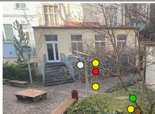
Situační umístění měřících zařízení: Vnitroblok Kodaňská-Estonská 3
